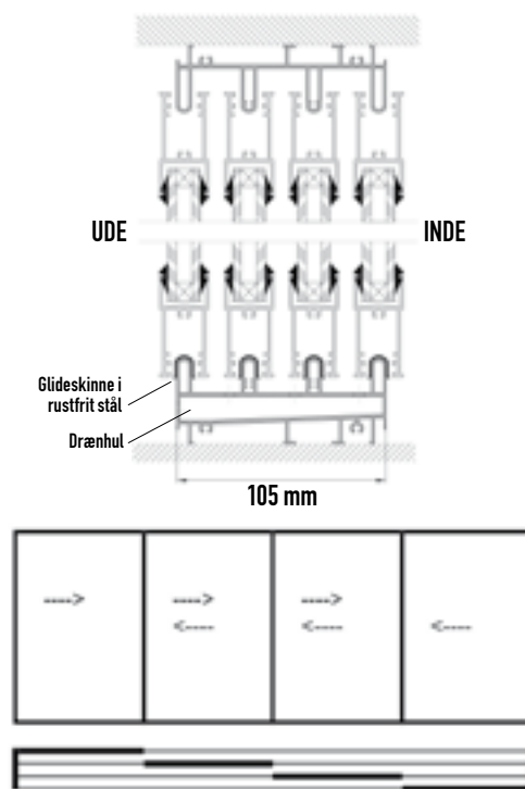
4 delt skydedør
